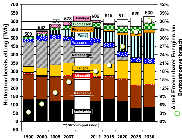
Abbildung 11: Referenzprognose Strombereitstellung
