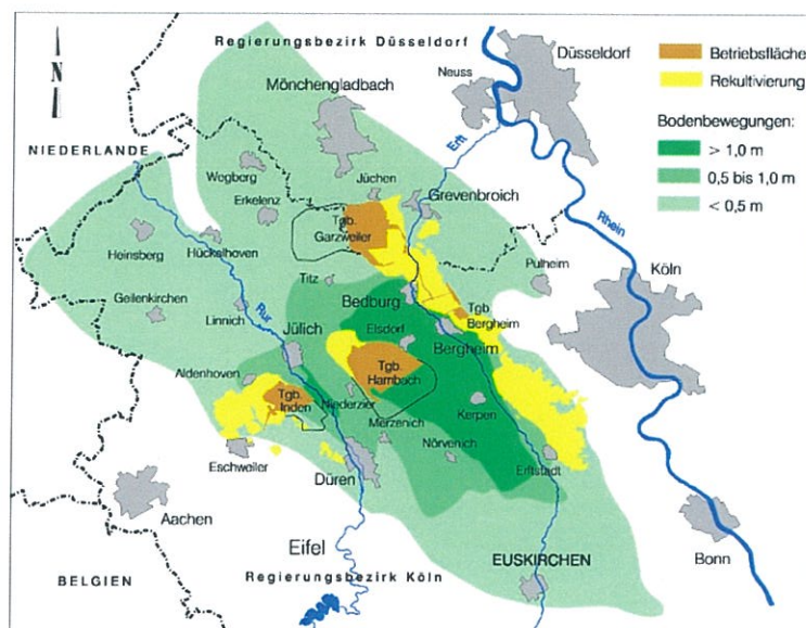
Abbildung 1: Überblick über die großräumigen Bodenbewegungen 1955 bis heute
